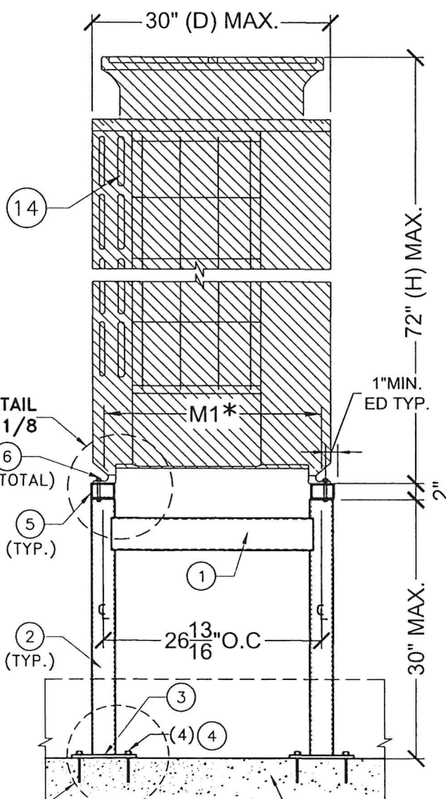
VIEW X SCALE: N.T.S.
