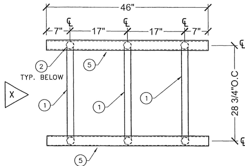
TYP. PLAN VIEW VRF STAND SCALE: N.T.S
